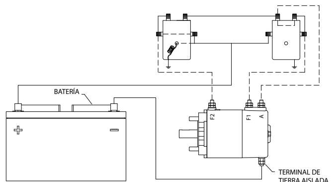
SOLENOIDES DE CONEXIONES DEL MOTOR
