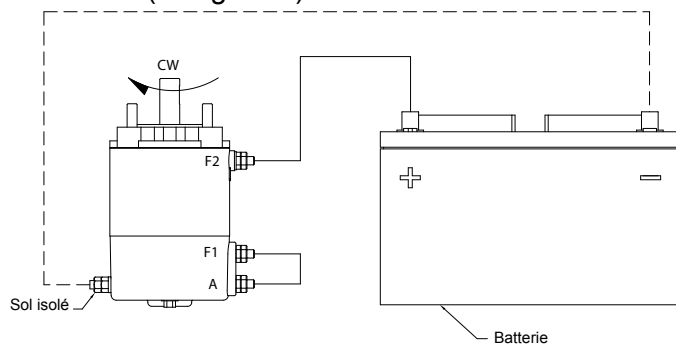
FIGURE-1 MOTEUR HORLOGE SAGE ROTATION
