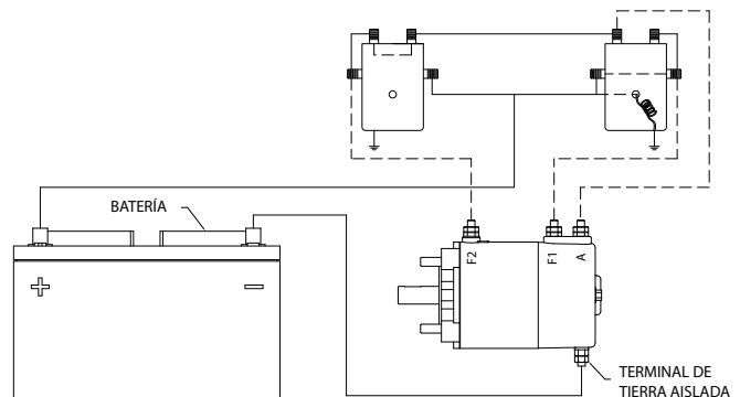
SOLENOIDES DE CONEXIONES DEL MOTOR
