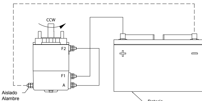
FIGURE-2 Motor - rotación a la derecha
