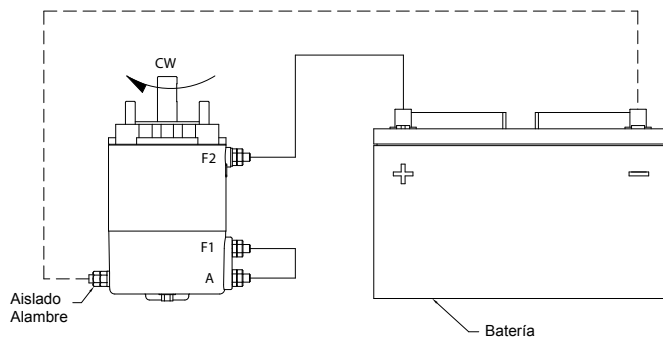
FIGURE-1 Motor - reloj contrario sabia rotación
